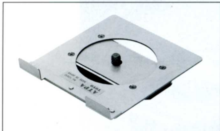
No.12032 マウンティングプレート45A・45A II用 ATPA このプレートは、QRC カメラオートクイックリリースに45A・45A IIをセットする際に使用します。
