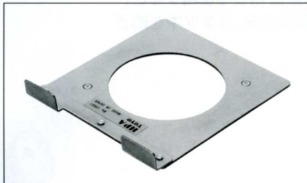
No.12031 雲台プレート 45A・45A II用 HPA トヨフィールド45A・45A IIと雲台(No.7501M-II)の間にはさみ、カメラが回転方向にズれるのを防ぎます。
