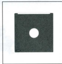
No.1601 LB4F 45A用標準ボード トヨフィールド45A用 標準レンズボード(0番穴あり) 110mm × 110mm
